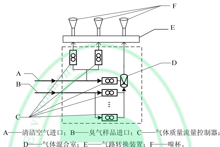
图 1 动态稀释嗅辨装置工作原理示意图
